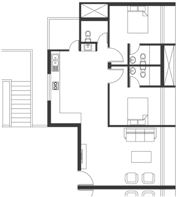
2-BHK UNIT
